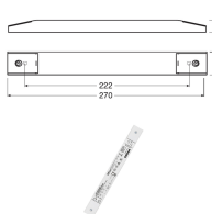
Caractéristiques Osram LED Driver Optotronic SLIM 30/220-240
